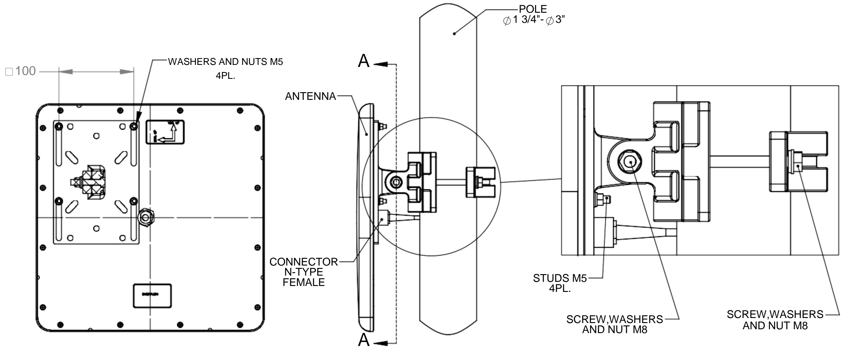
SECTION A-A
